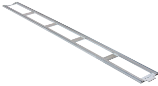
TRO-0475-13-00-00-0 Ansamblu cale rulare 1800 mm (70,9") Distanța dintre centrele ghidajelor în V" 152 mm (6")
