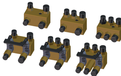
UCW-0475-59-00-00-0 Suport precis pentru fixare torță automată \phi 30mm (1.18")
